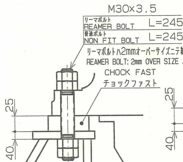
機関据付ボルト SETTING BOLT FOR MAIN ENGINE
