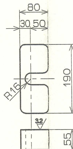
中間軸軸受用チョクライナー CHOCK LINER FOR INTERM.SHAFT BEARING
